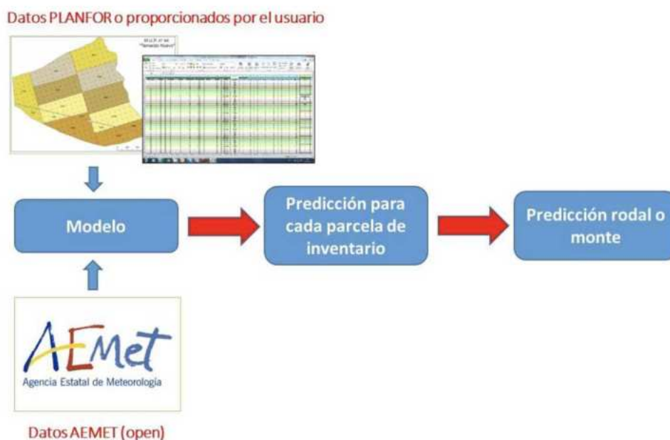
Figura 1. Esquema de flujo de la aplicación PINEA ClimaDAT
